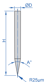
cone stylus (profile)
