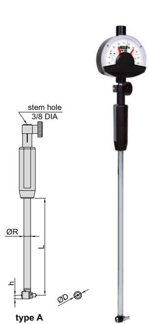
2435-E201
